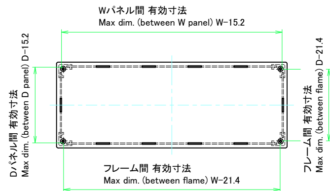
下カバー / Bottom cover
